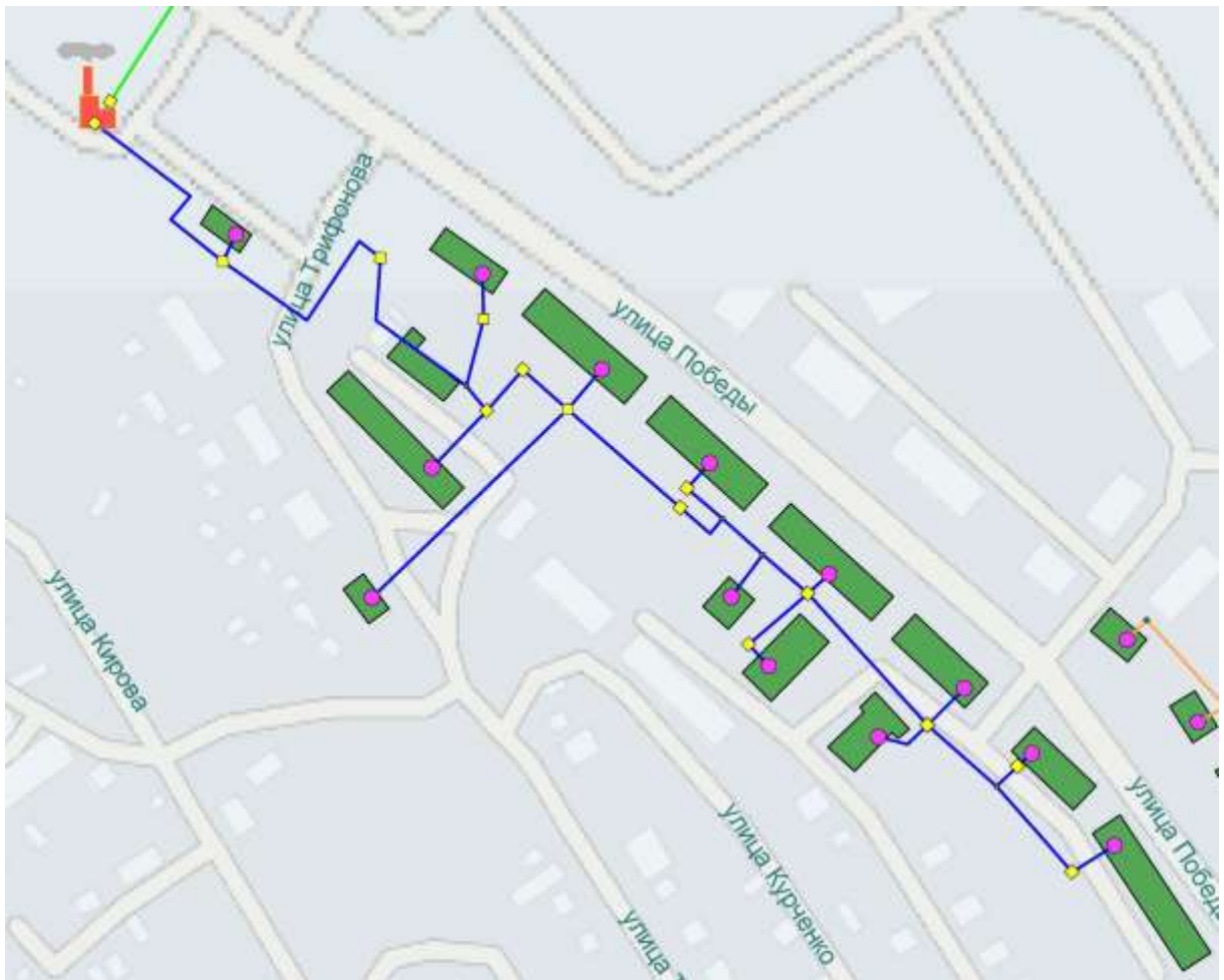
Рисунок 110. Участки предлагаемые к реконструкции.
