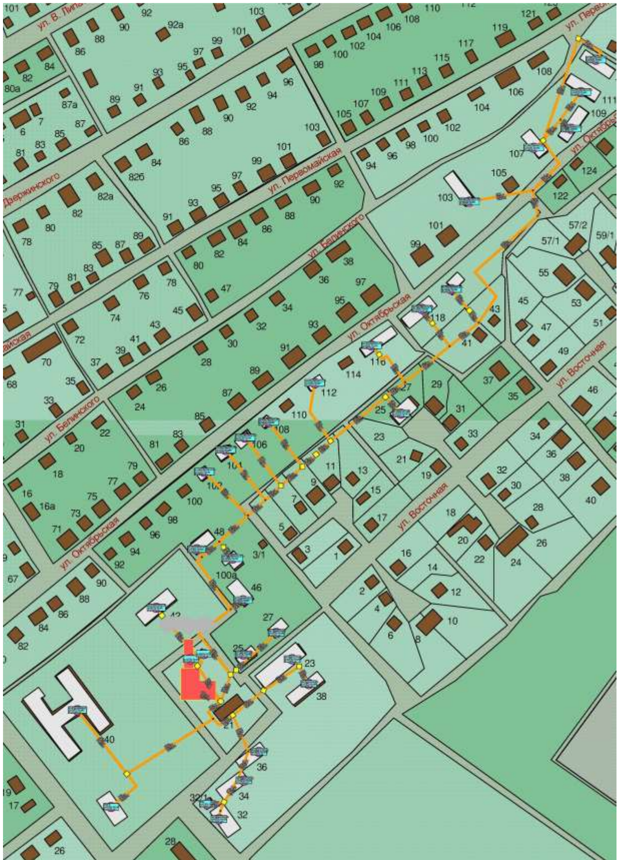
Рисунок 98. Зона действия котельной «Школьная».
