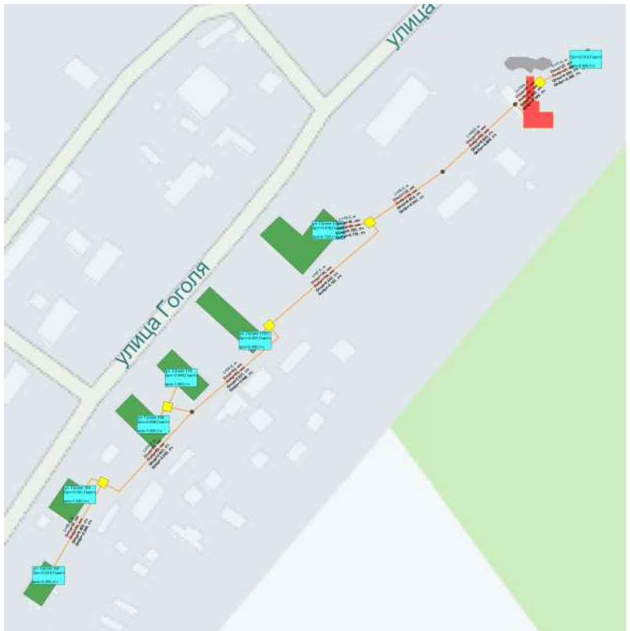
Рисунок 85. Зона действия котельной «Феникс».
