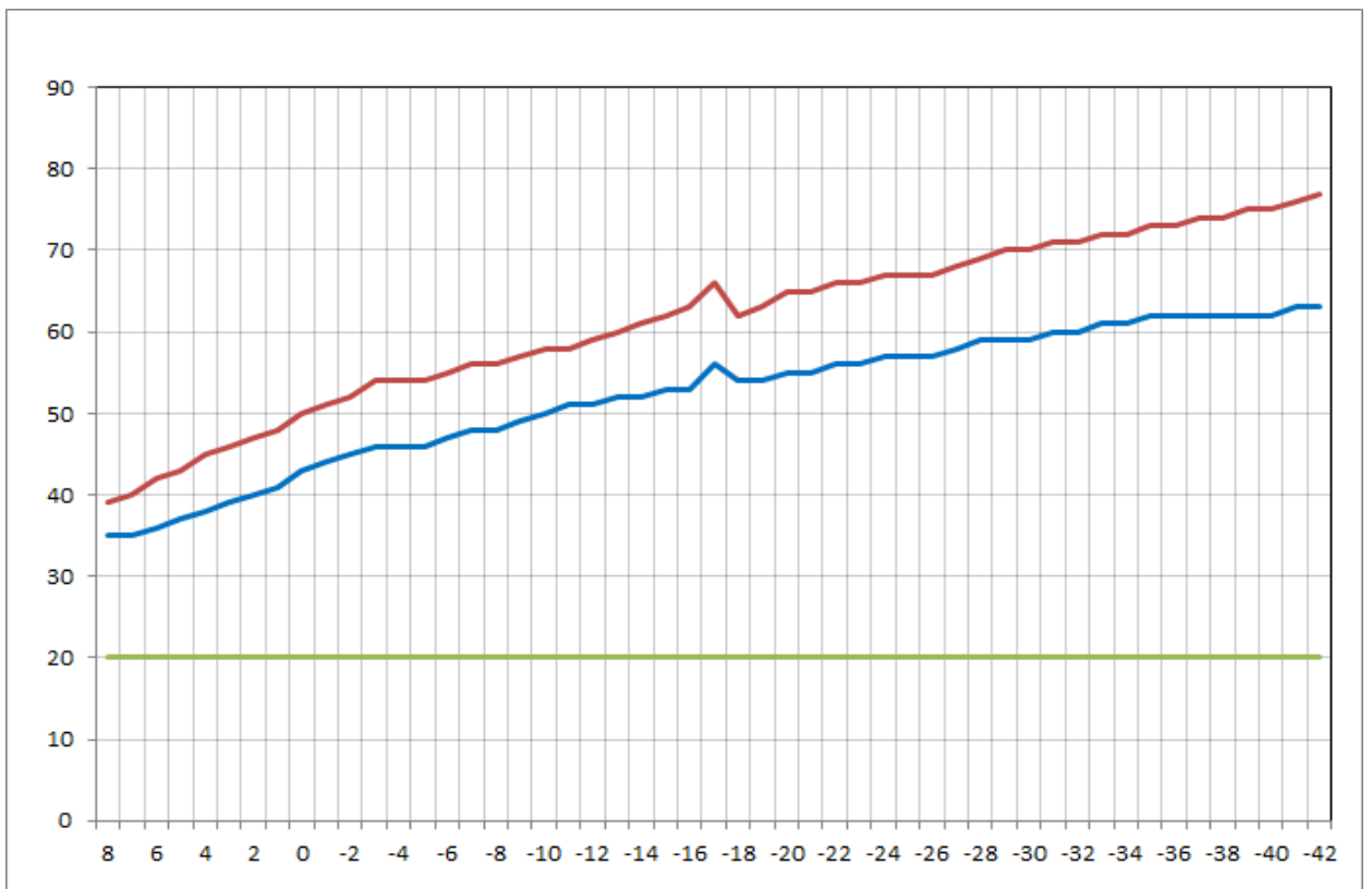
Рисунок 53. График регулирования температуры котельной «Лазо».
