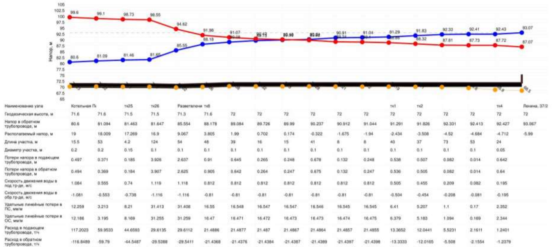
Пьезометрический график от котельной «Педучилище» до самого удаленного потребителя.
