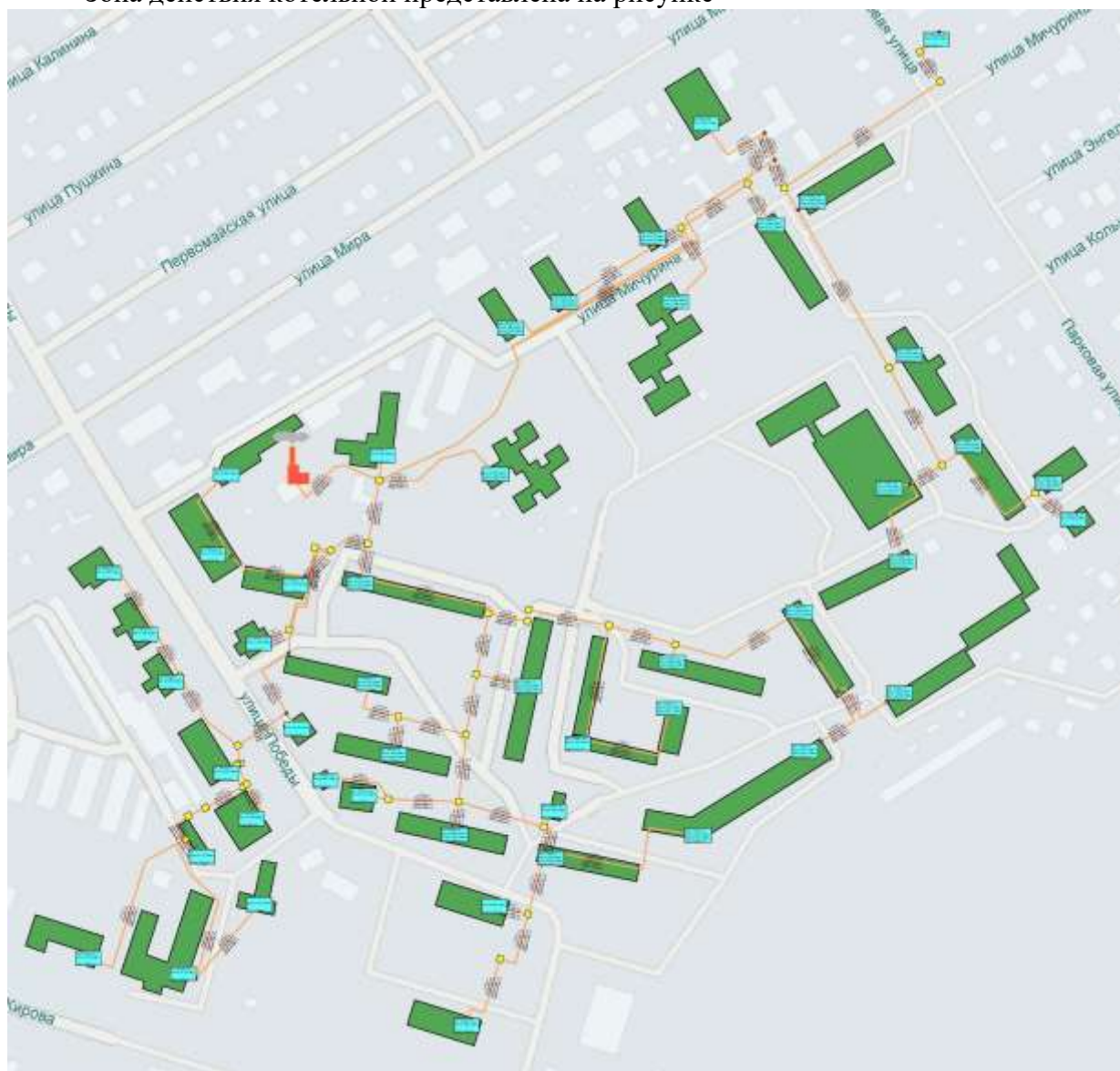
Рисунок 83. Зона действия котельной «Геолог».
