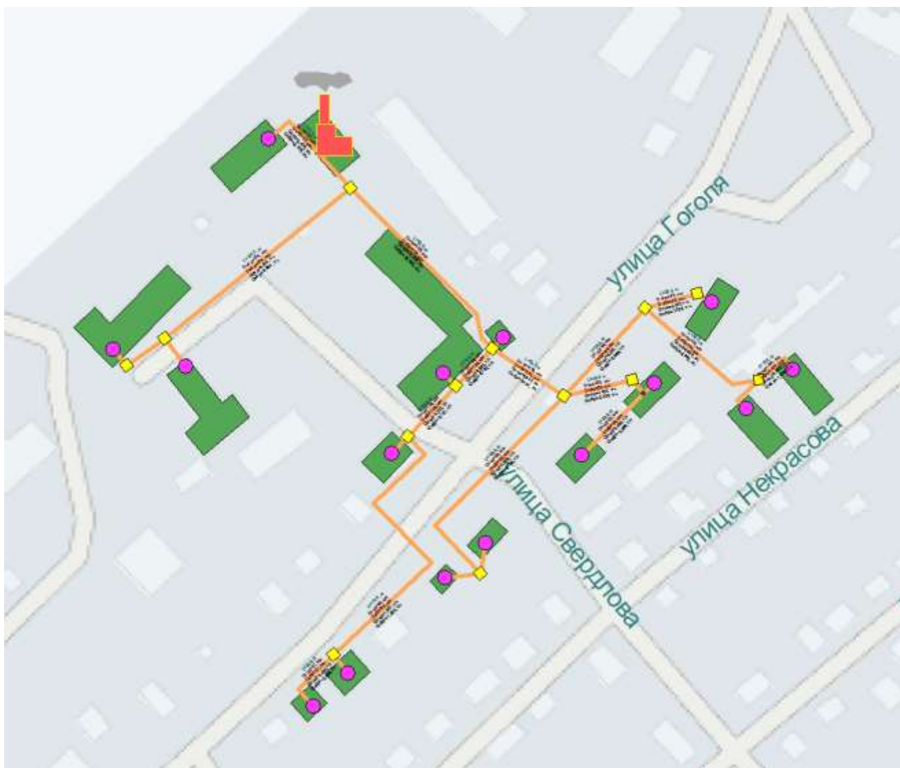
Рисунок 47. Схема тепловых сетей котельной «ДРСУ».
