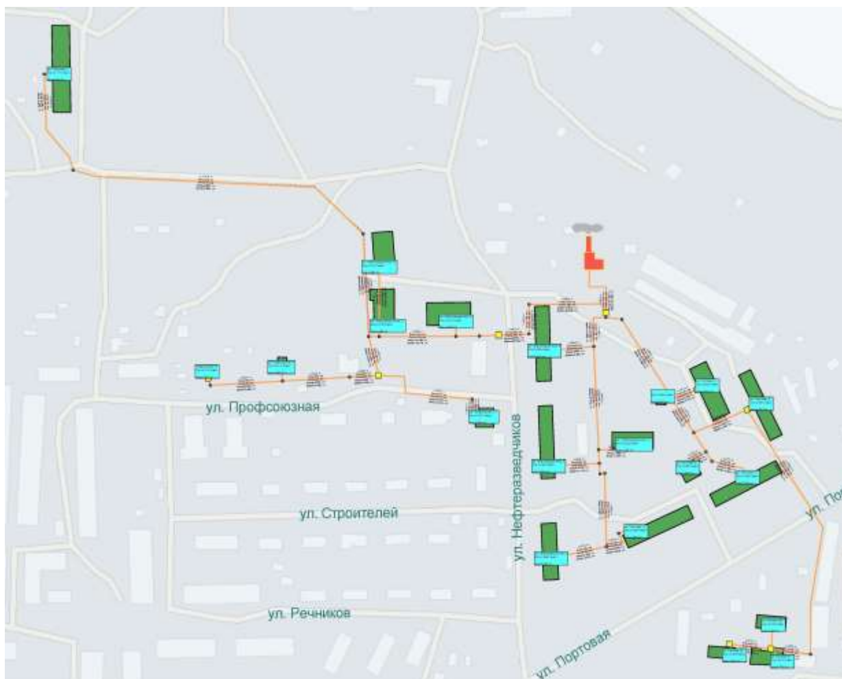
Рисунок 84. Зона действия котельной «КОНГРЭ».
