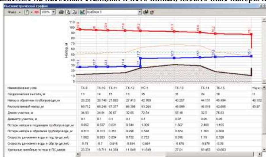
Рисунок 120. Пьезометрический график.
