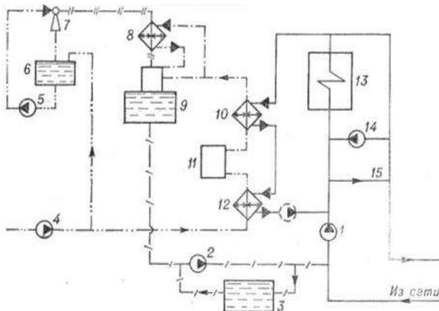
1—сетевой насос; 2—подпиточный насос; 3—бак подпиточной воды; 4—насос исходной воды; 5—насос подачи воды к эжектору; 6—расходный бак эжекторной установки; 7—водоструйный эжектор; 8—охладитель пара; 9—вакуумный деаэрактор; 10—подогреватель химически очищенной воды; 11—фильтр химводоочистки; 12—подогреватель исходной воды; 13—водогрейный котел; 14—рециркуляционный насос; 15—линия перепуска.
