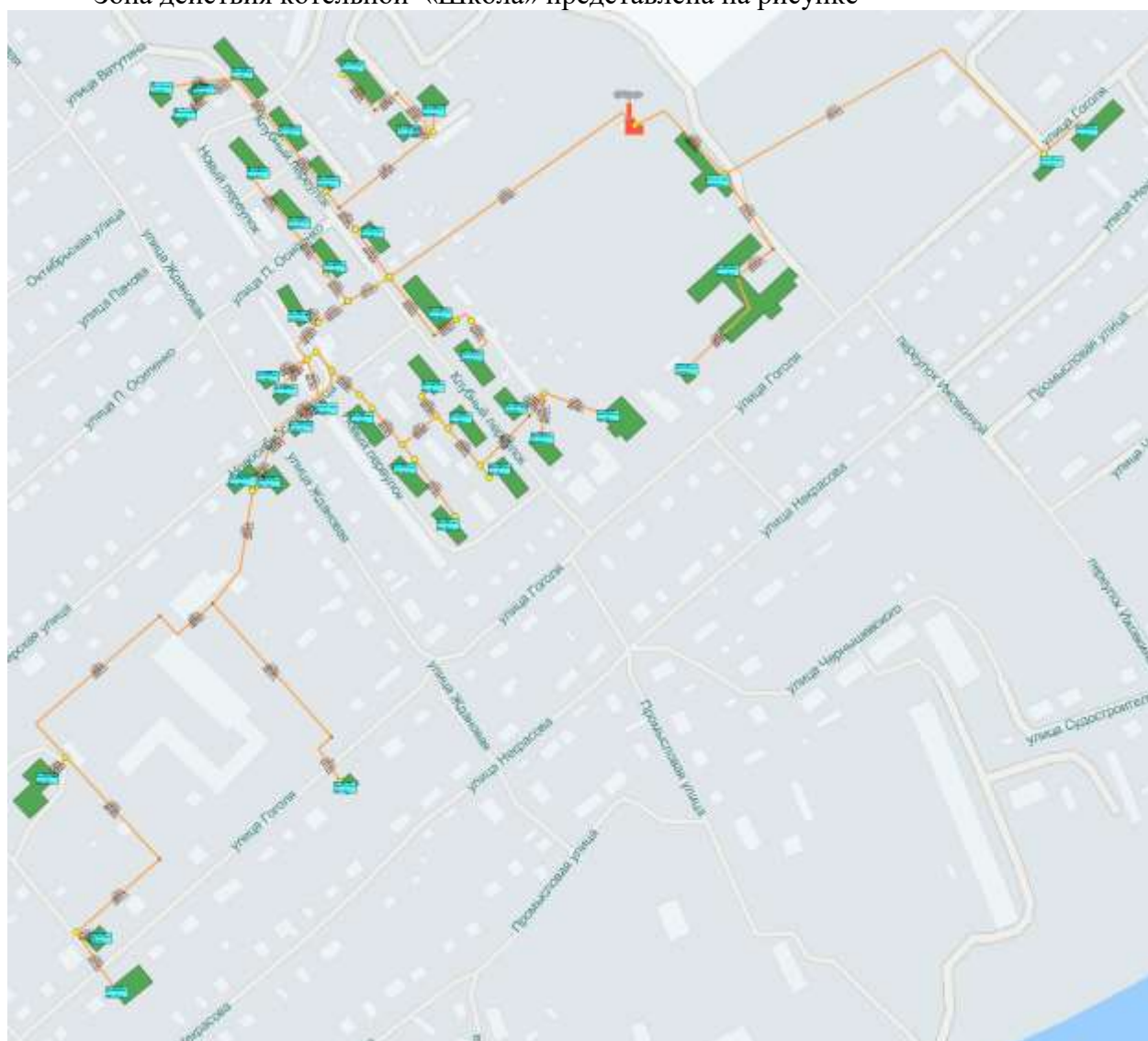
Рисунок 82. Зона действия котельной «Школа».
