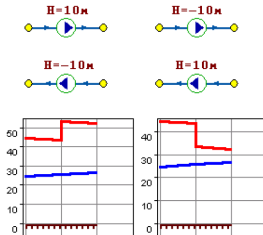
Рисунок 116. Пьезометрические графики.
