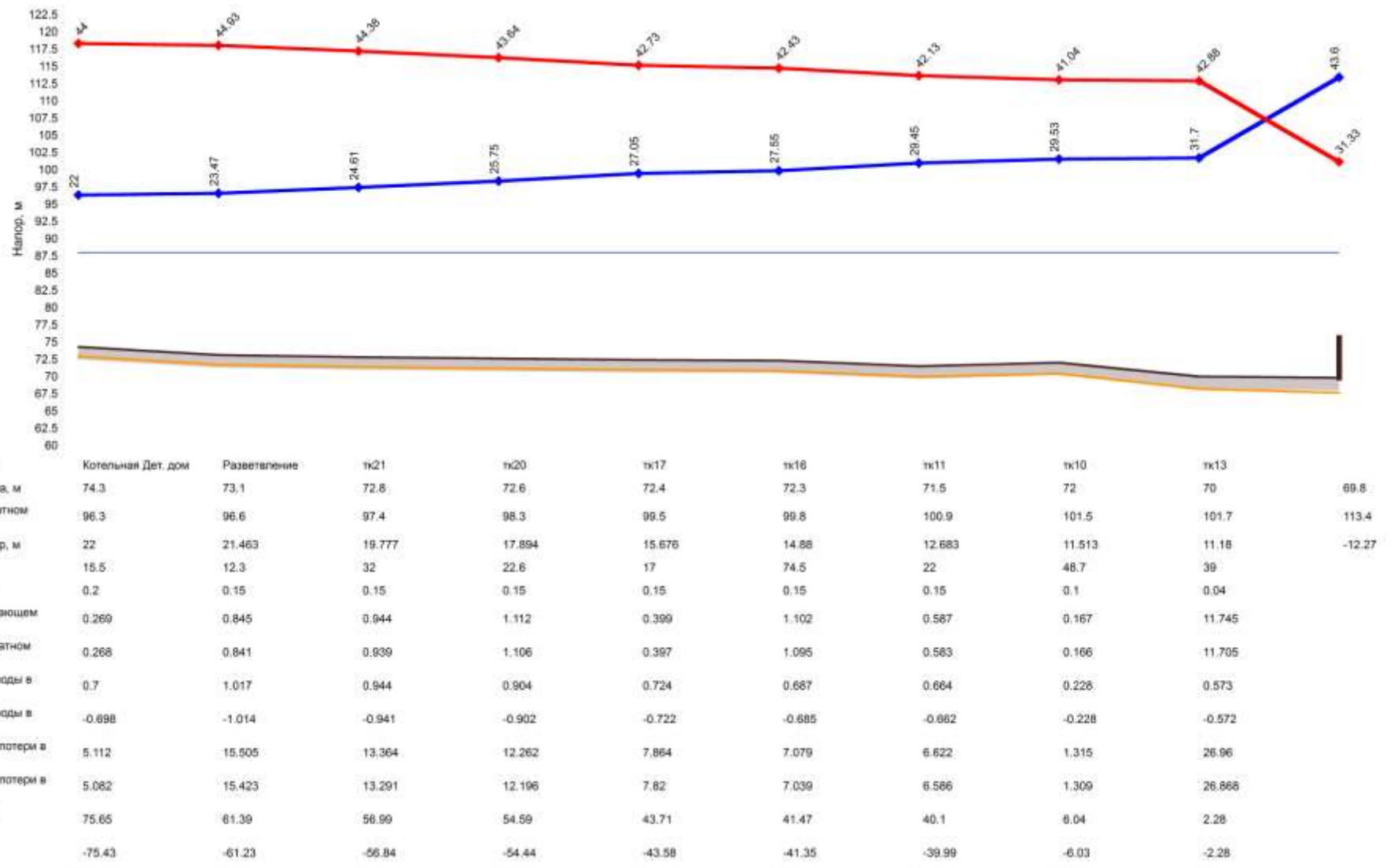
Рис. 69 Пьезометрический график от котельной «Детский дом» до жилого дома по адресу ул. Некрасова 2.
