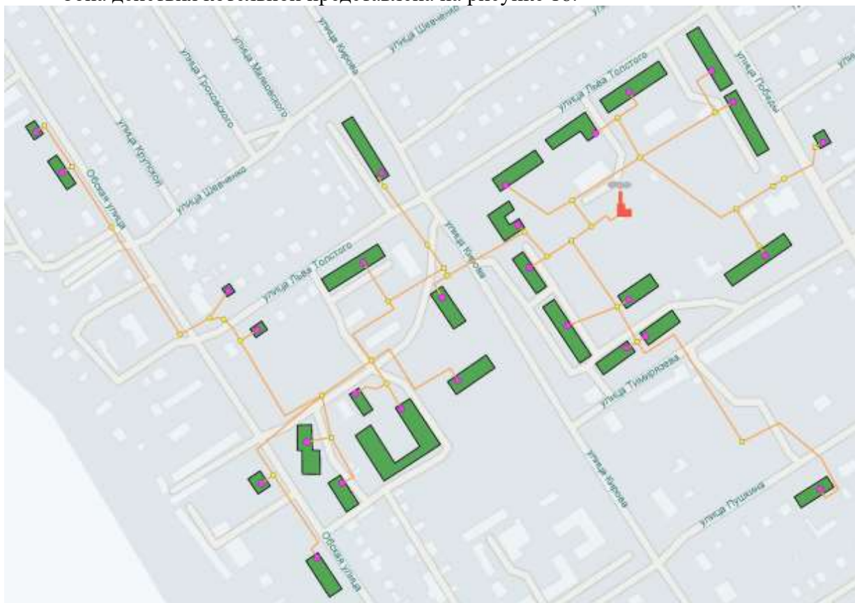
Рисунок 17. Зона действия котельной «Победы».
