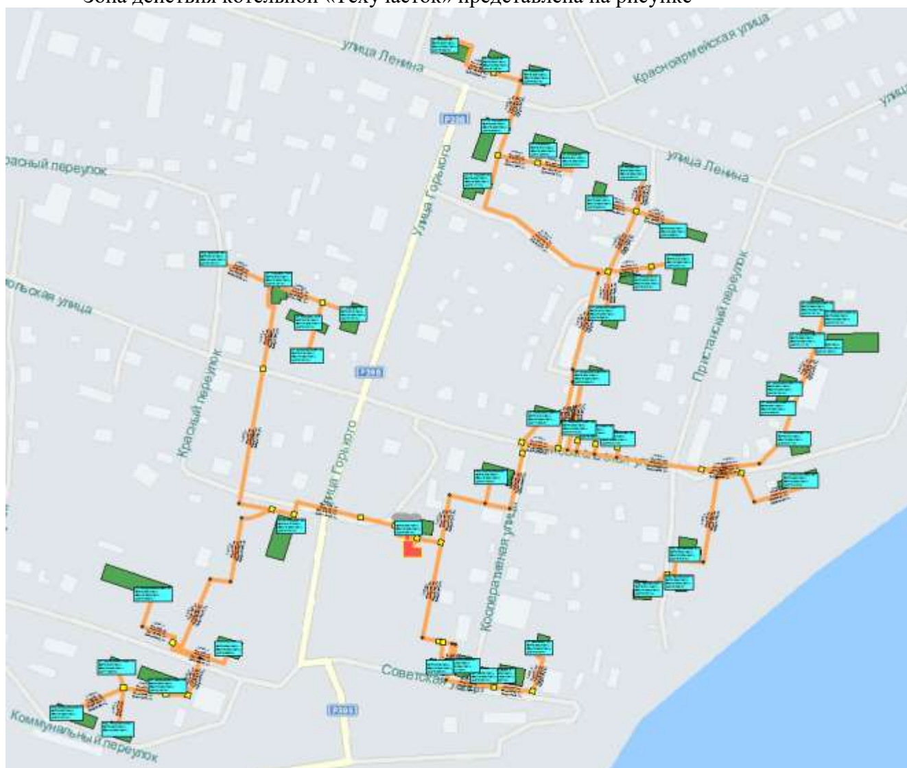
Рисунок 80. Зона действия котельной «Техучасток».
