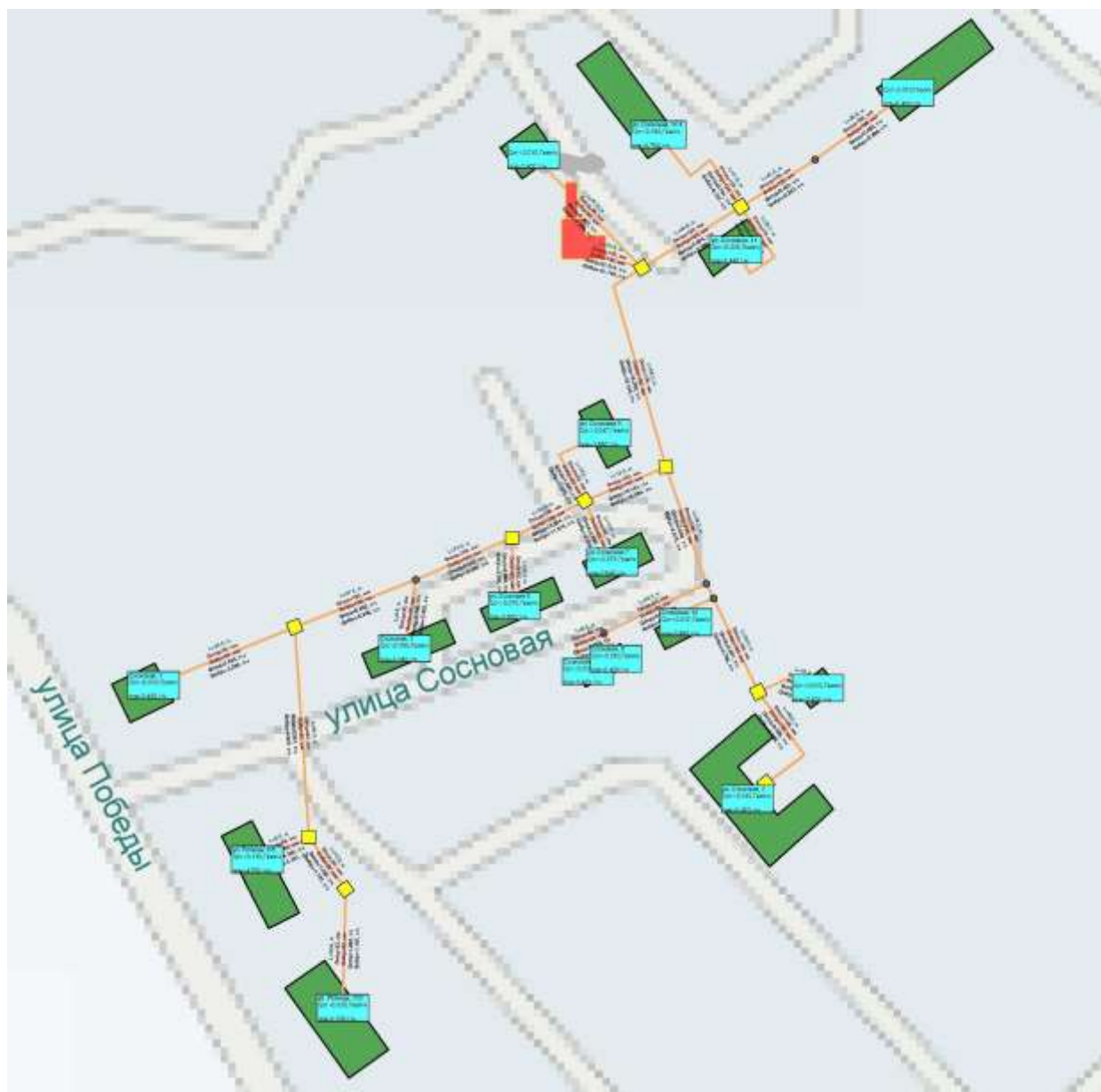
Рисунок 81. Зона действия котельной «Урожай».
