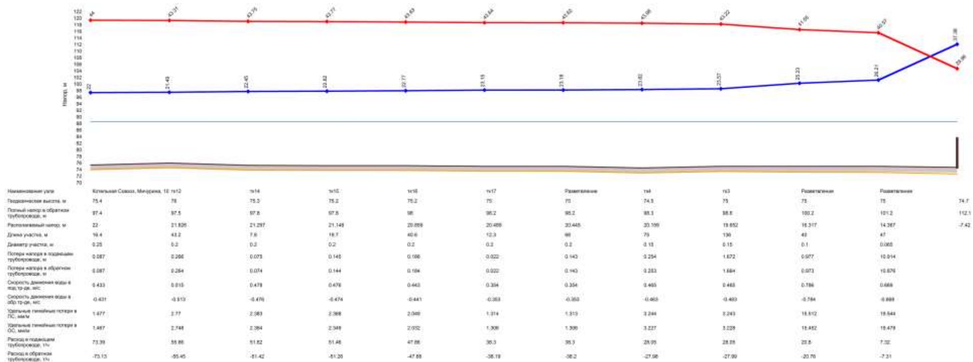
Рис. 71 Пьезометрический график от котельной «Совхозная» до жилого дома по адресу ул. Сибирская 3.
