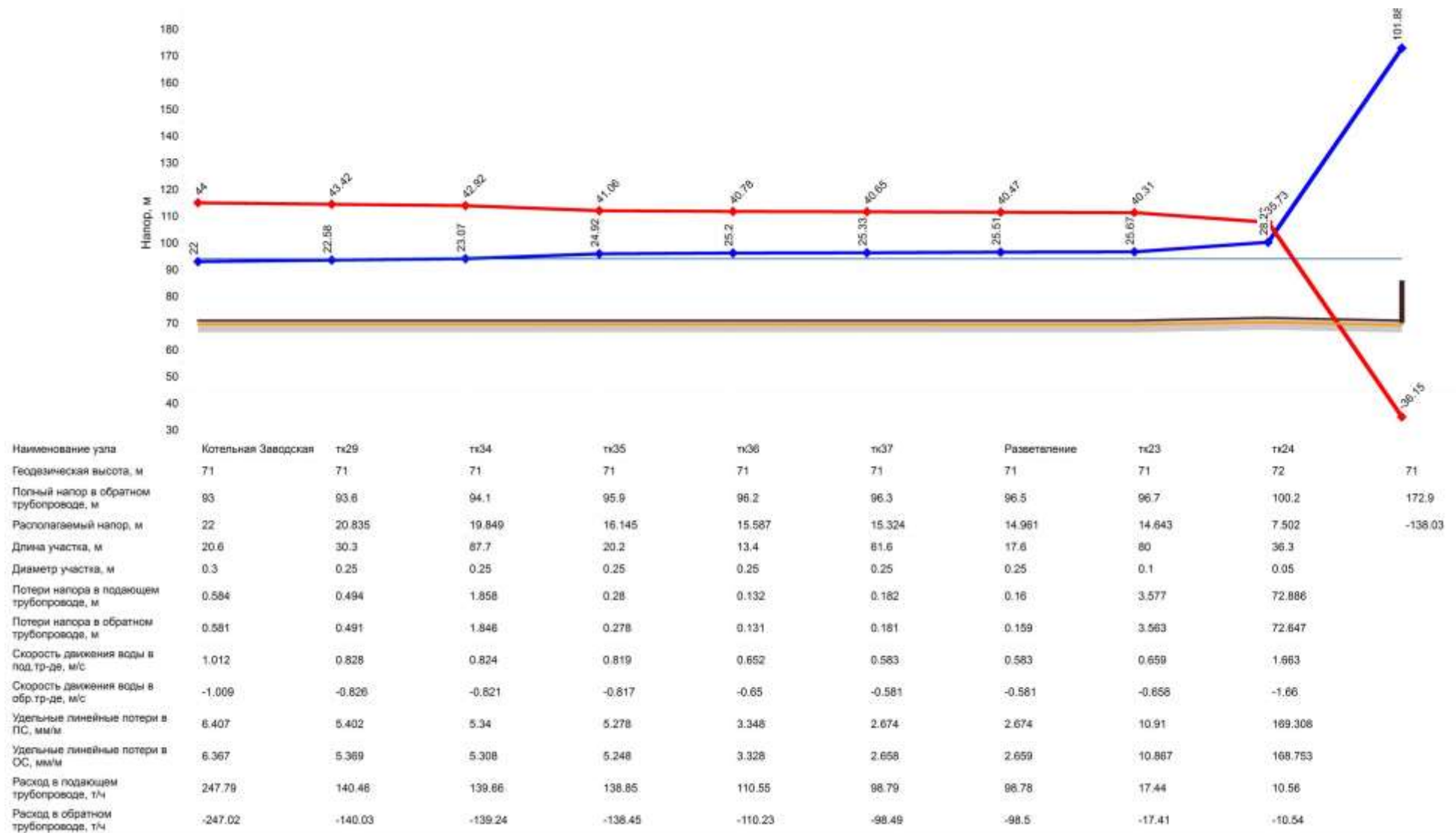
Рис. 72 Пьезометрический график от котельной «Совхозная» до жилого дома по адресу ул. Свердлова 5
