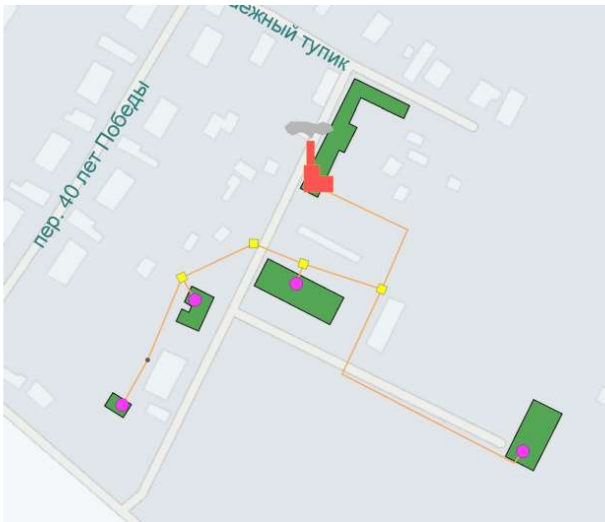
Рисунок 28. Схема тепловых сетей котельной «Телецентр».
