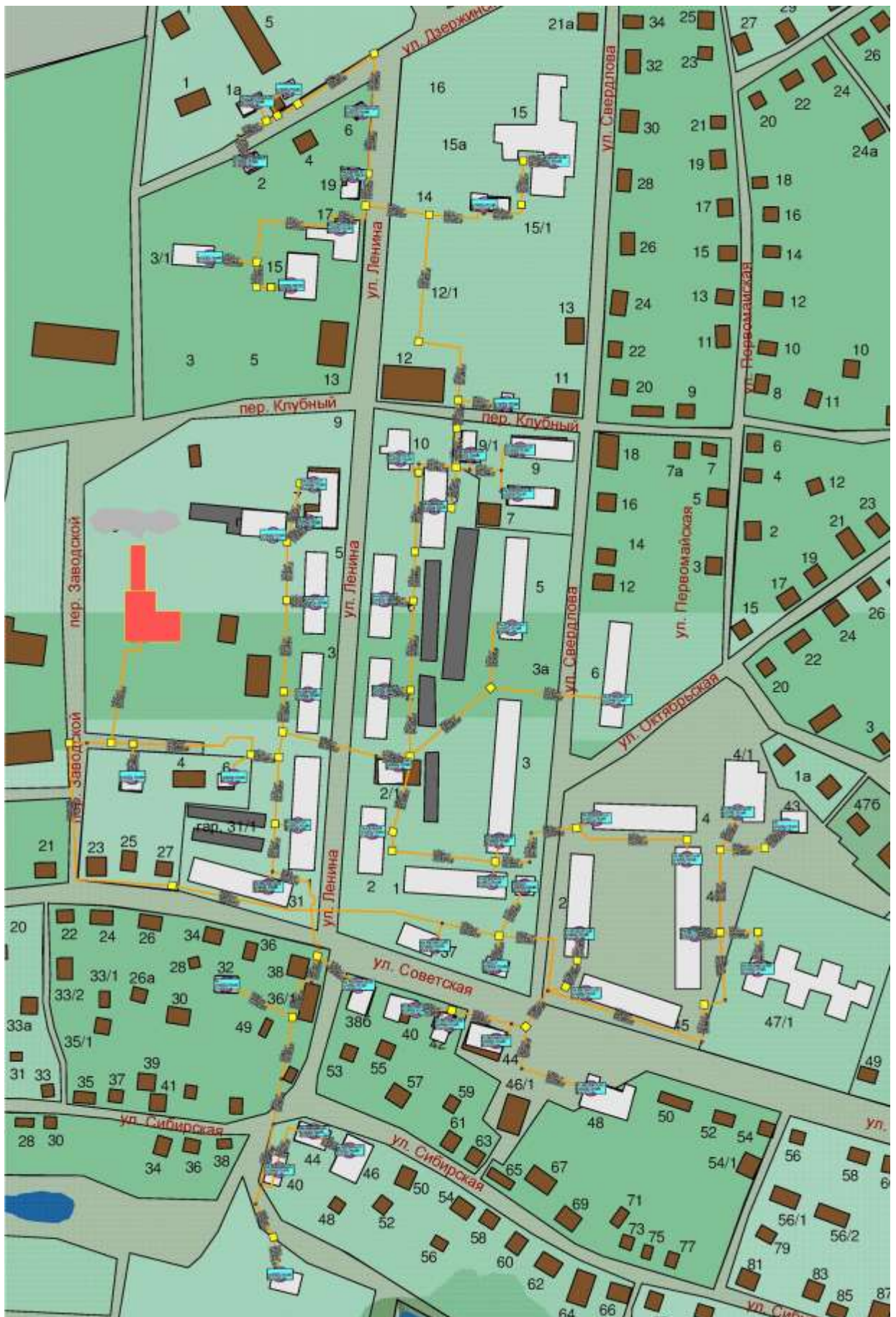
Рисунок 96. Зона действия котельной «Заводская».
