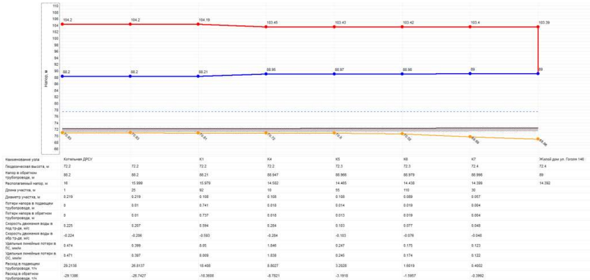
Рис. 74 Пьезометрический график от котельной «ДРСУ» до дома по улице Гоголя 146.
