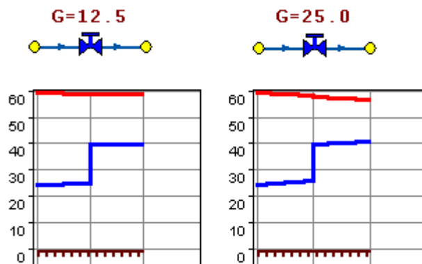
Рисунок 119. Регулятор давления.
