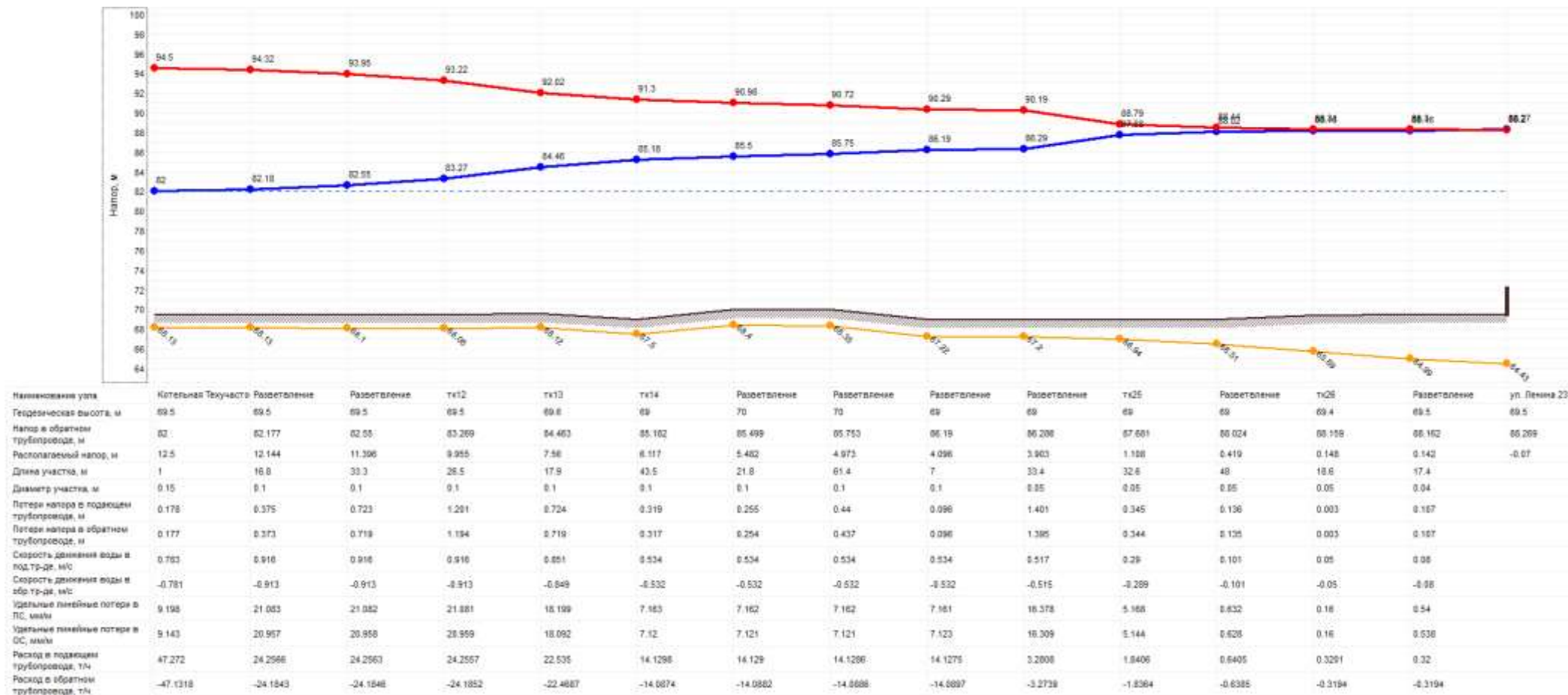
Рис. 56 Пьезометрический график от котельной «Техучасток» до жилого дома по адресу ул. Ленина 23.
