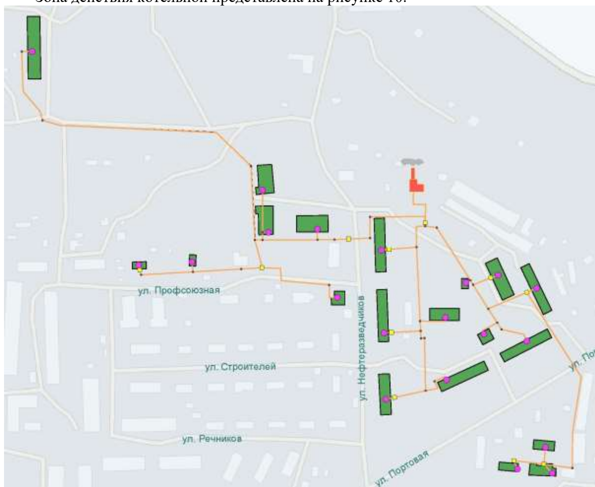
Рисунок 9. Зона действия котельной «КОНГРЭ».
