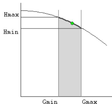
Рисунок 117. Напорно-расходная характеристика насоса.
