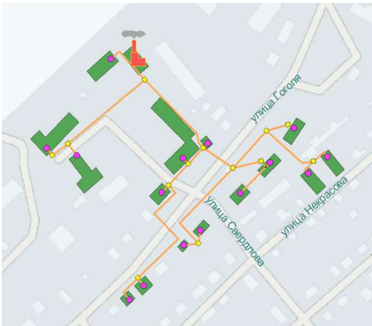
Рисунок 23. Зона действия котельной «ДРСУ».
