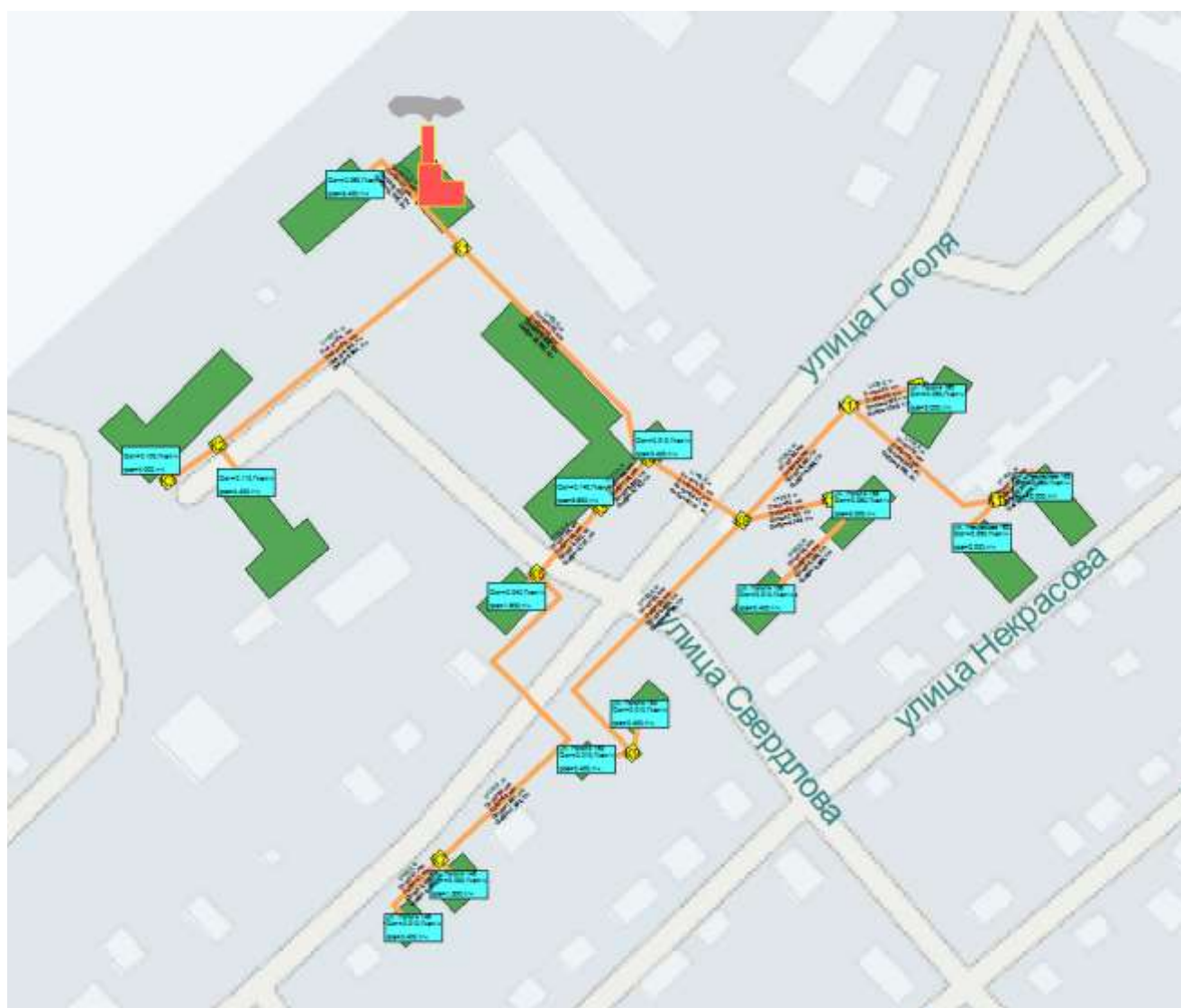
Рисунок 98. Зона действия котельной «ДРСУ».
