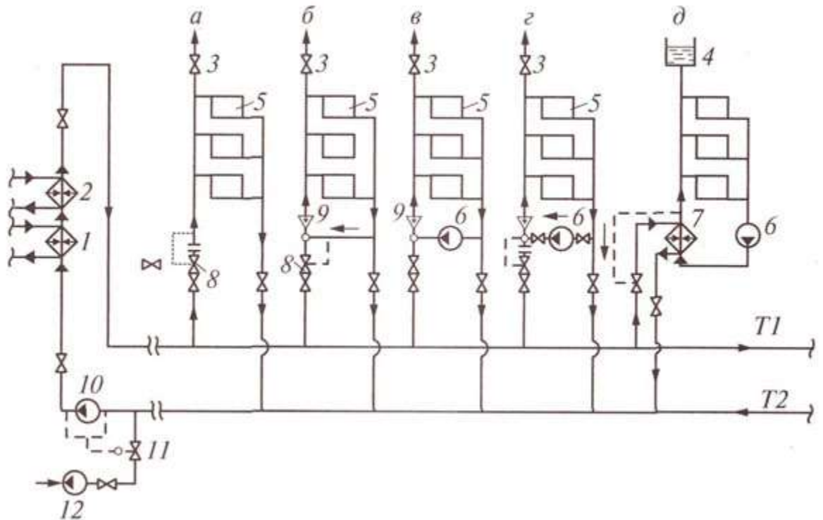
Рисунок 75. Тепловой узел.
