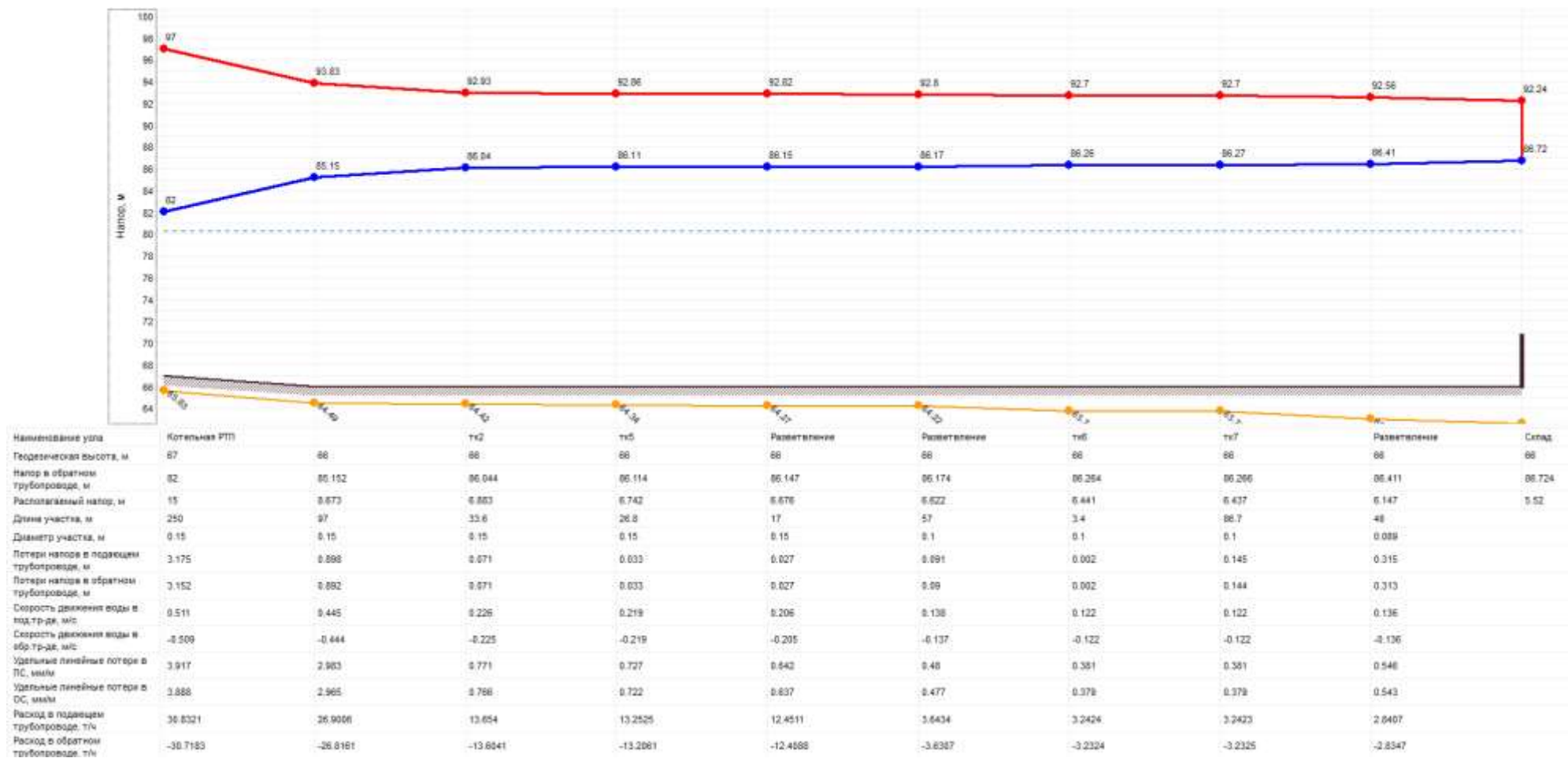
Рис. 65 Пьезометрический график от котельной «РТП» до жилого дома по адресу ул. Обская 93/1.
