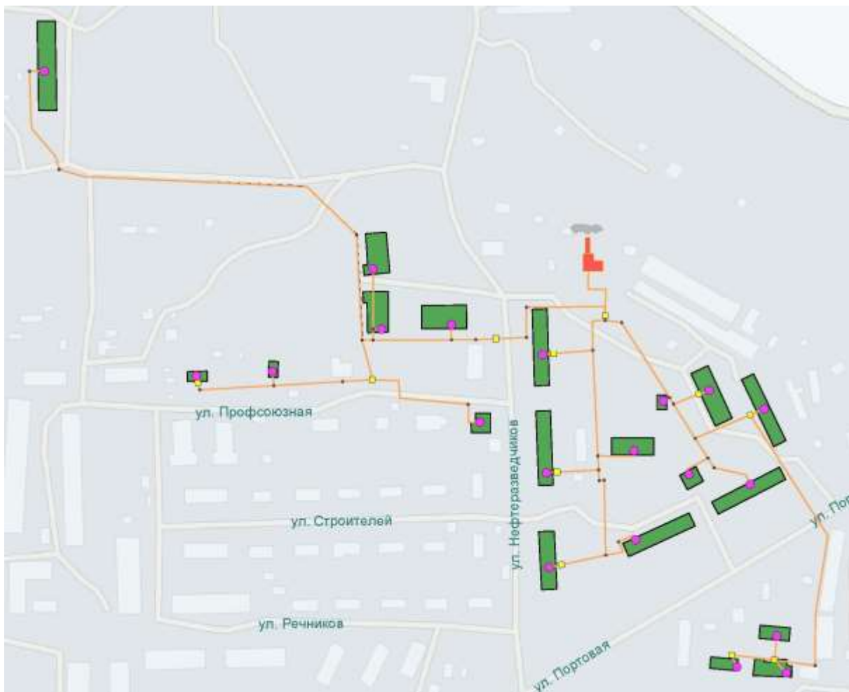
Рисунок 33. Схема тепловых сетей котельной «КОНГРЭ».
