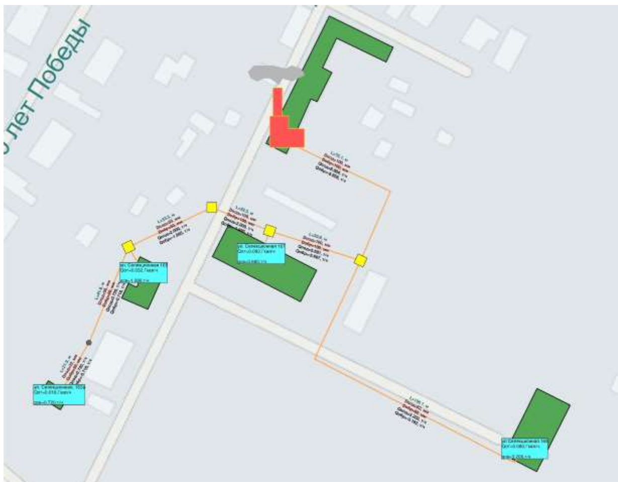
Рисунок 79. Зона действия котельной «Телецентр».
