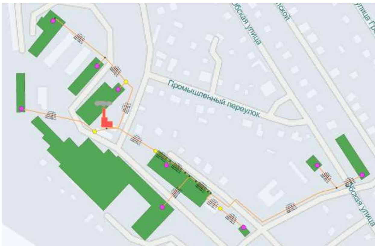
Рисунок 46. Схема тепловых сетей котельной «Металлист».
