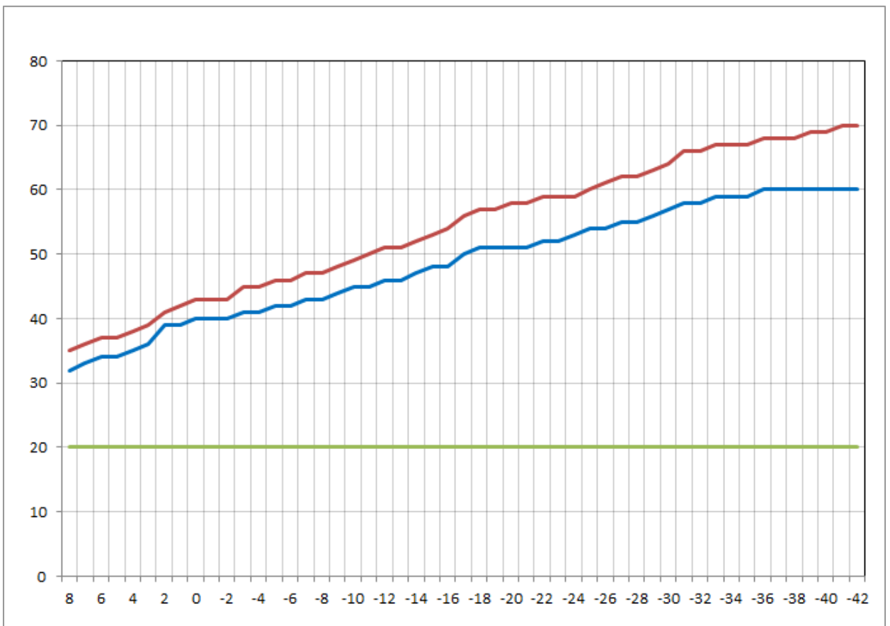
Рисунок 51. График регулирования температуры угольных котельных, находящихся в ведении МУП «Пламя».
