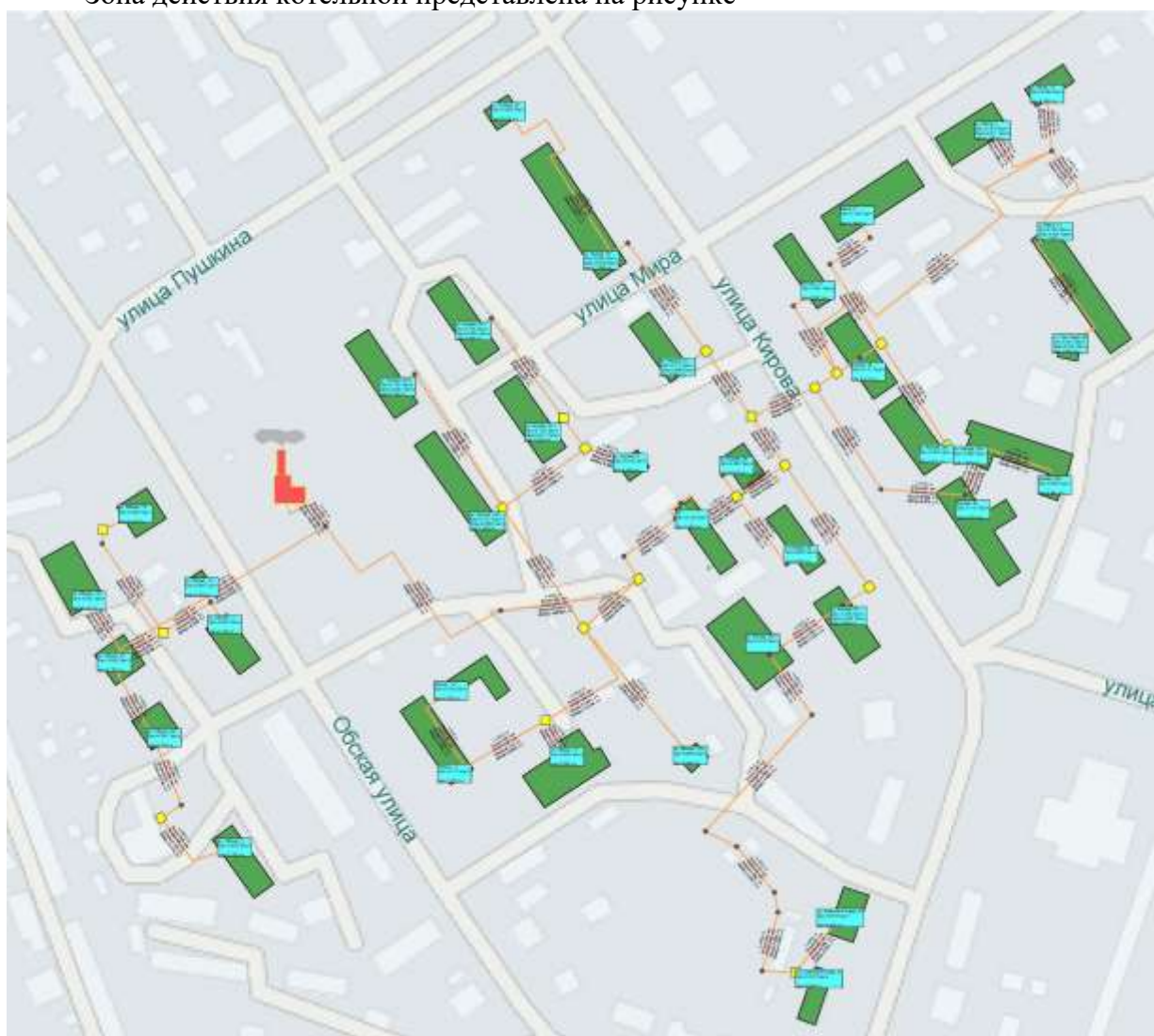
Рисунок 87. Зона действия котельной «ДПО».
