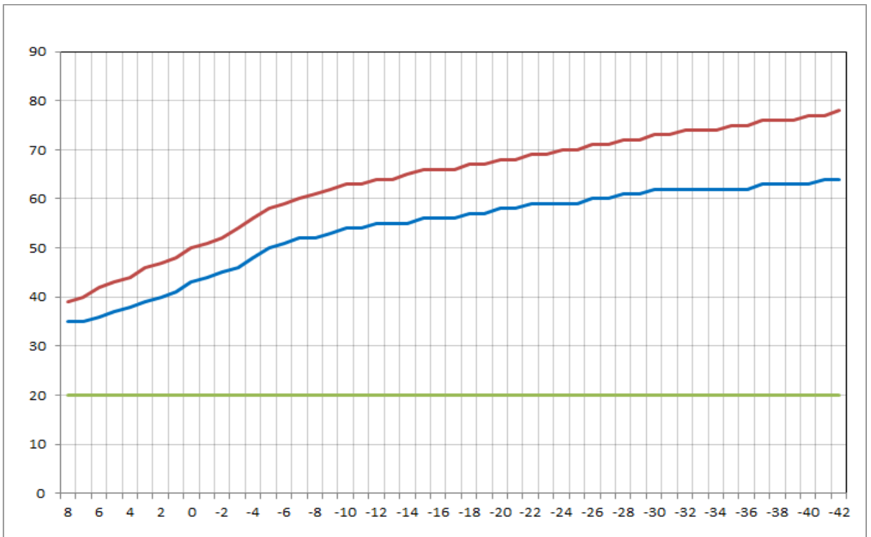
Рисунок 48. График регулирования температуры котельных «Звезда», «Школа» и «Урожай».
