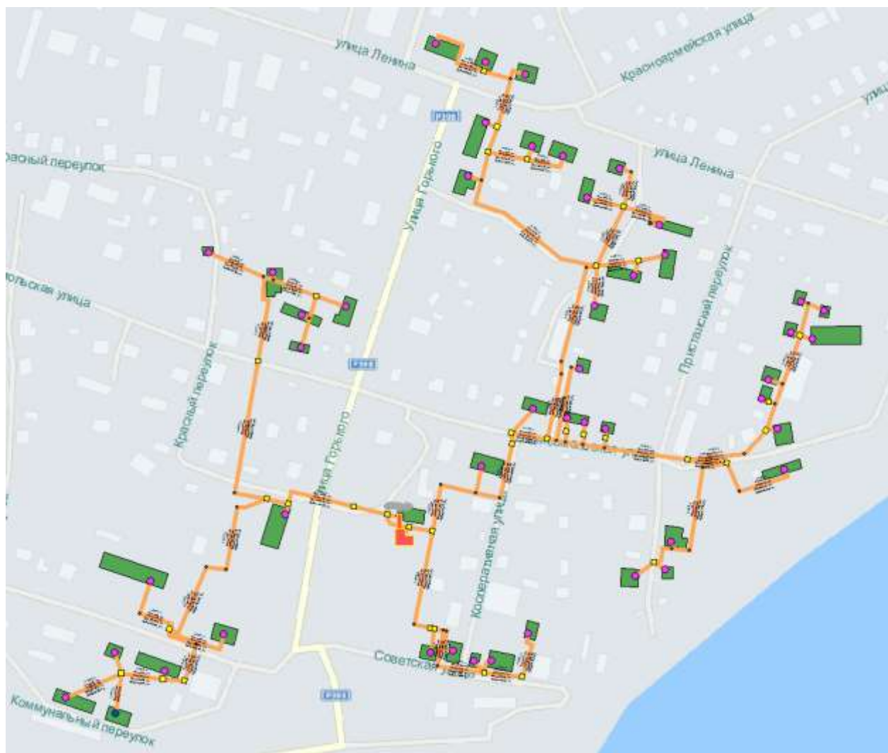
Рисунок 29. Схема тепловых сетей котельной «Техучасток».
