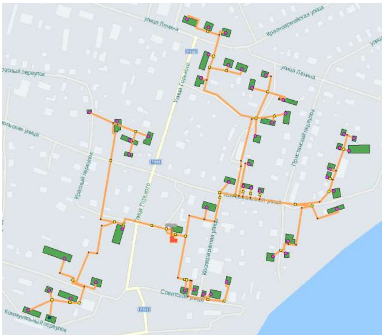
Рисунок 5. Зона действия котельной «Техучасток».
