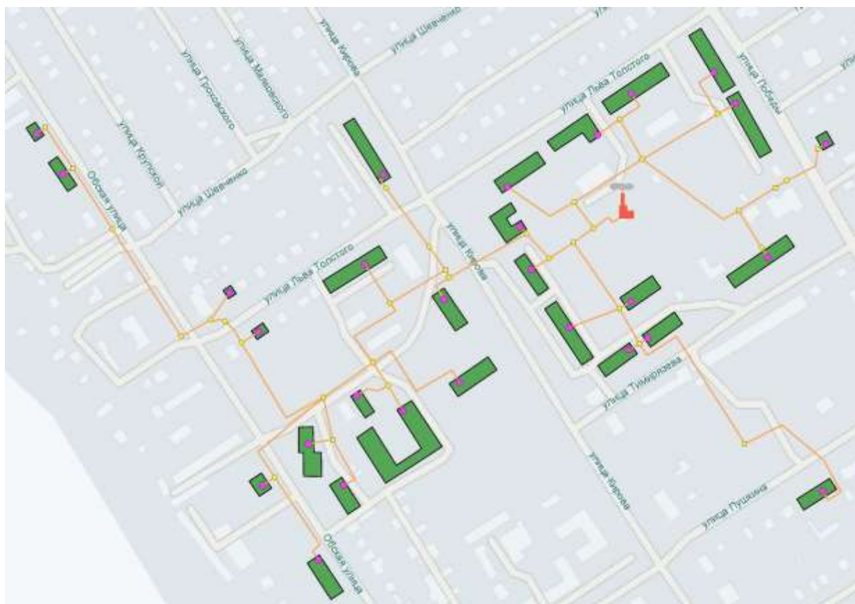
Рисунок 41. Схема тепловых сетей котельной «Победы».
