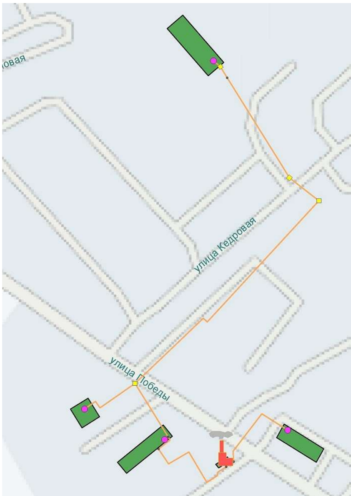
Рисунок 15. Зона действия котельной «РММ».
