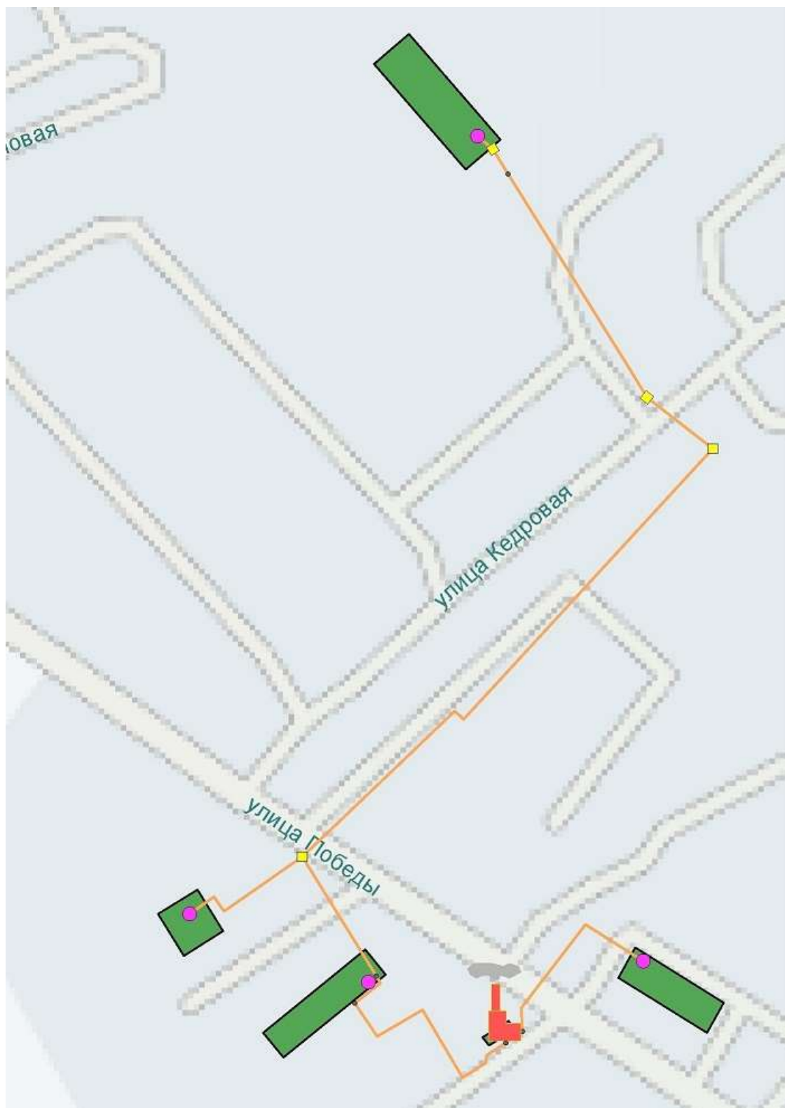
Рисунок 39. Схема тепловых сетей котельной «РММ».
