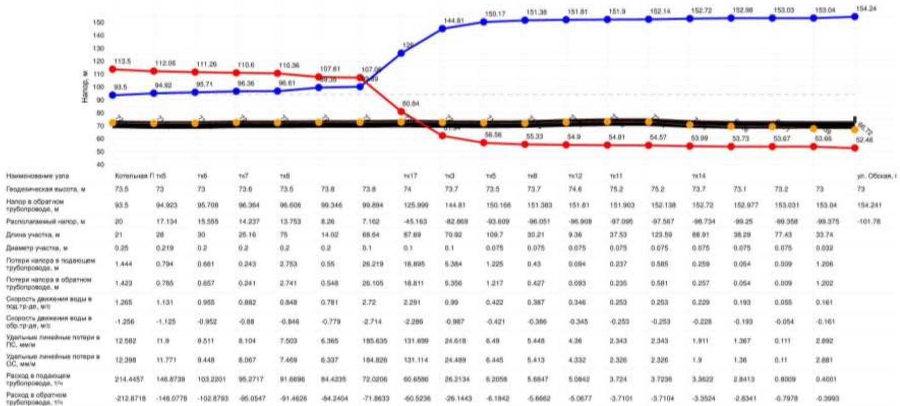
Пьезометрический график от котельной «Победы» до самого удаленного потребителя.
