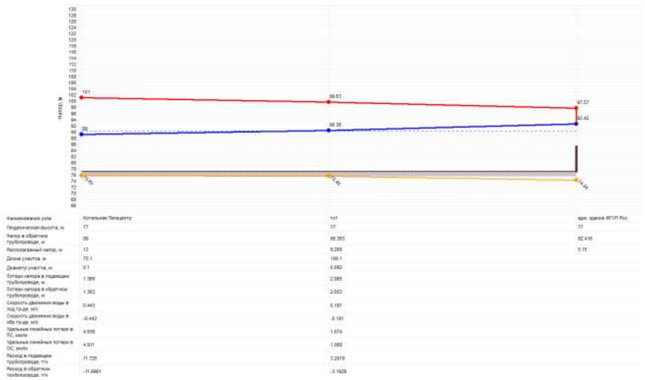
Рис. 56 Пьезометрический график от котельной «Телецентр» до административного здания ФГУП.
