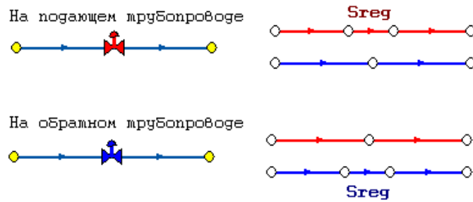
Рисунок 135. Дросселирующие устройства.
