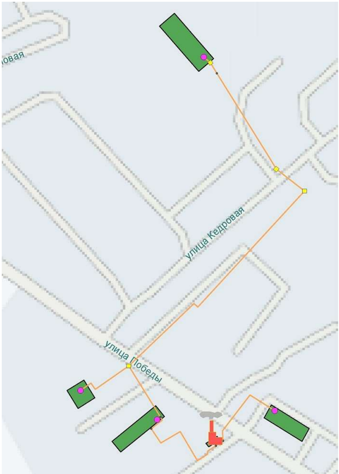
Рисунок 16. Зона действия котельной «РММ».
