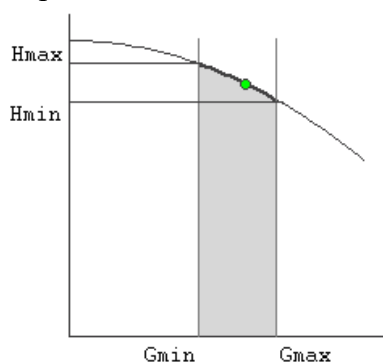
Рисунок 134. Напорно-расходная характеристика насоса.
