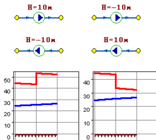
Рисунок 133. Пьезометрические графики.
