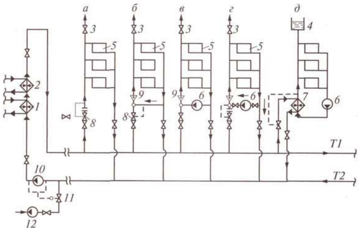
Рисунок 78. Тепловой узел.
