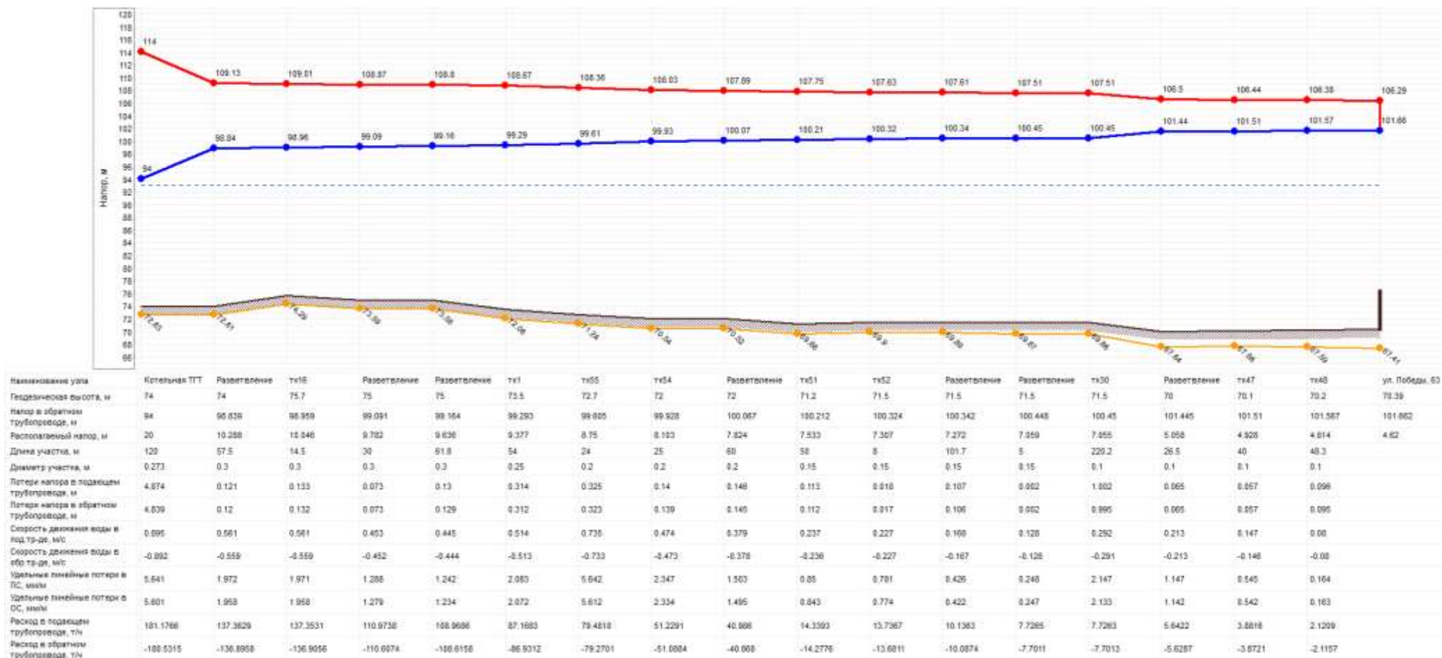
Пьезометрический график от котельной «ТГТ» до самого удаленного потребителя.
