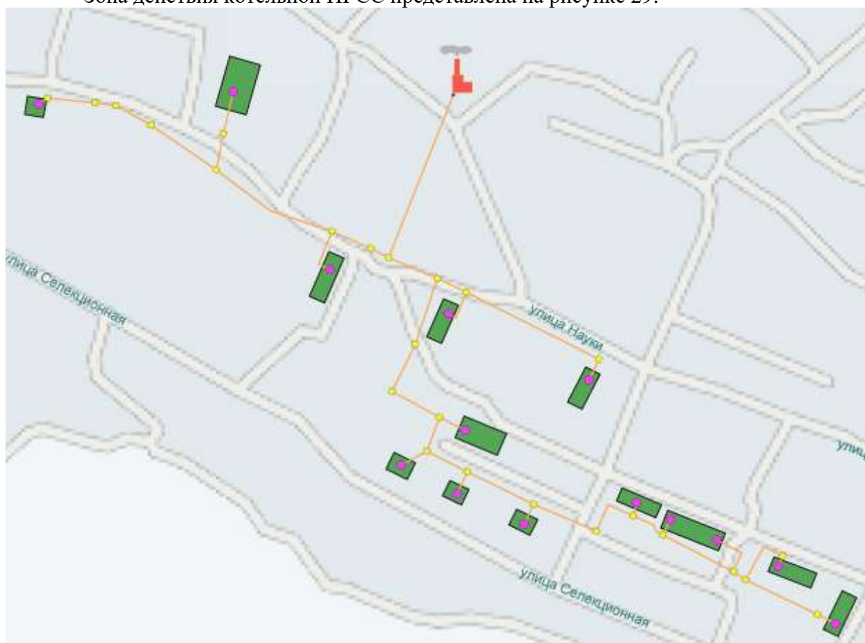
Рисунок 29. Схема тепловых сетей котельной НГСС.
