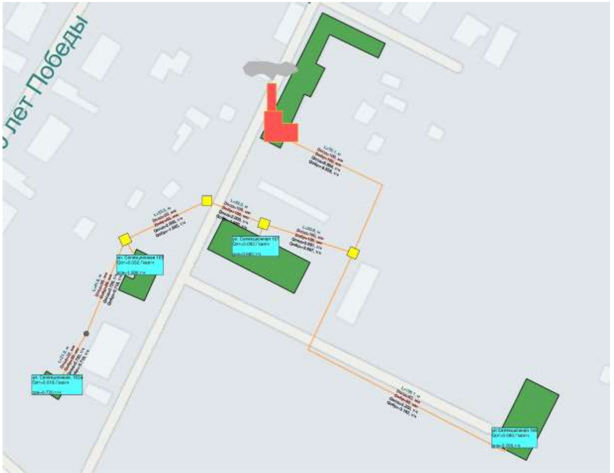
Рисунок 82. Зона действия котельной «Телецентр».
