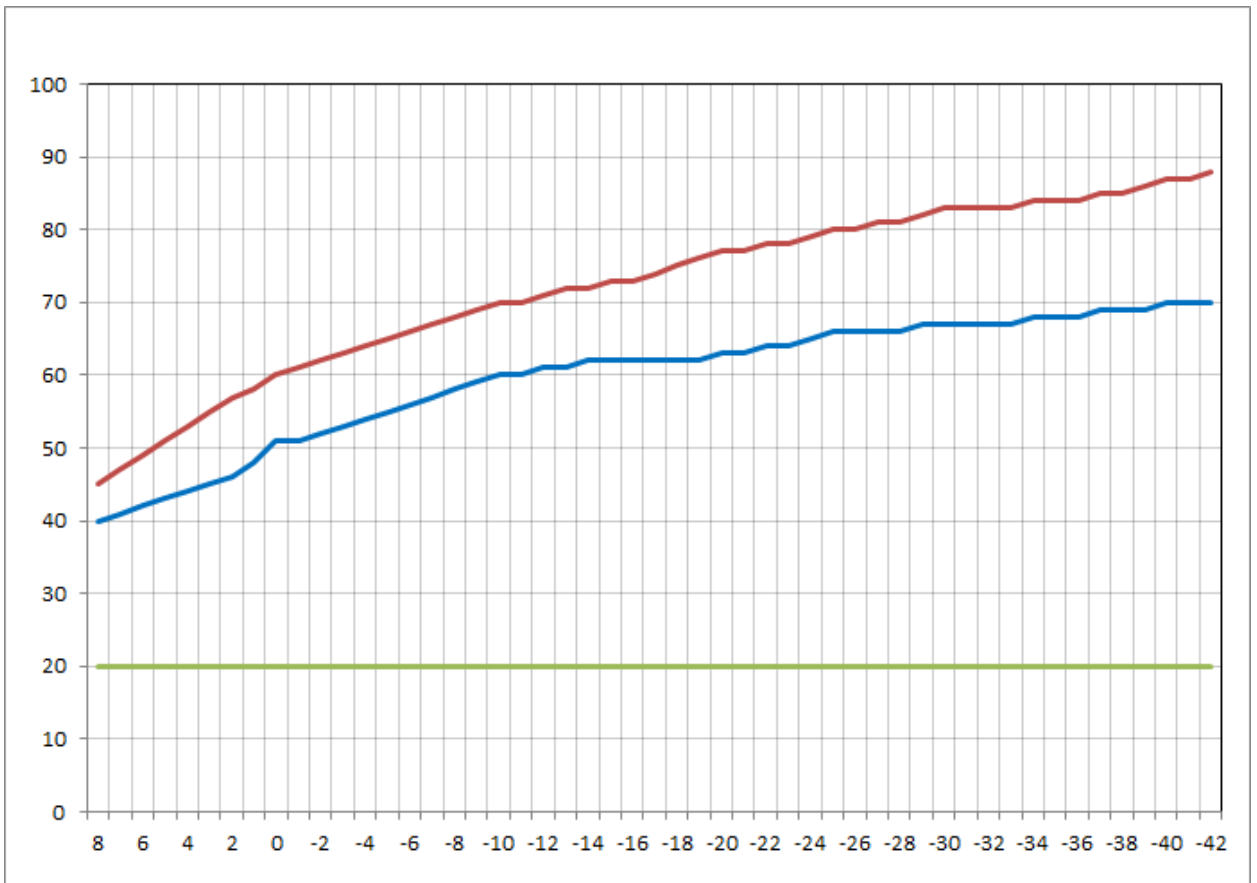
Рисунок 54. График регулирования температуры котельной «Техучасток».
