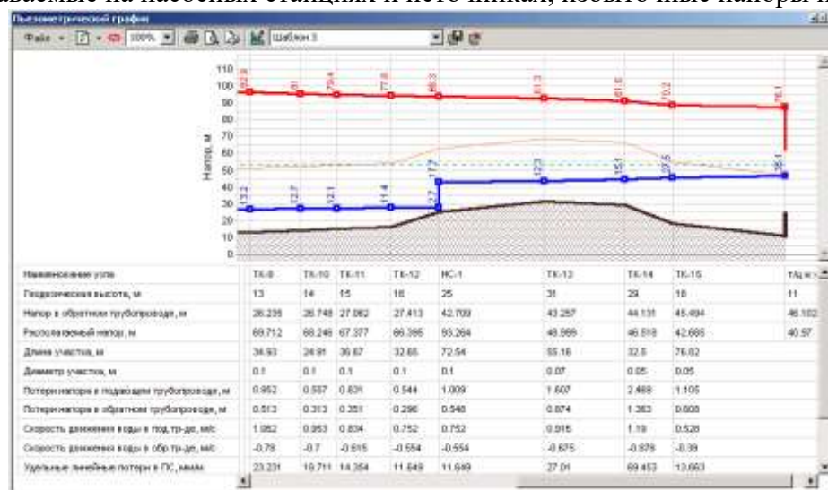
Рисунок 138. Пьезометрический график.
