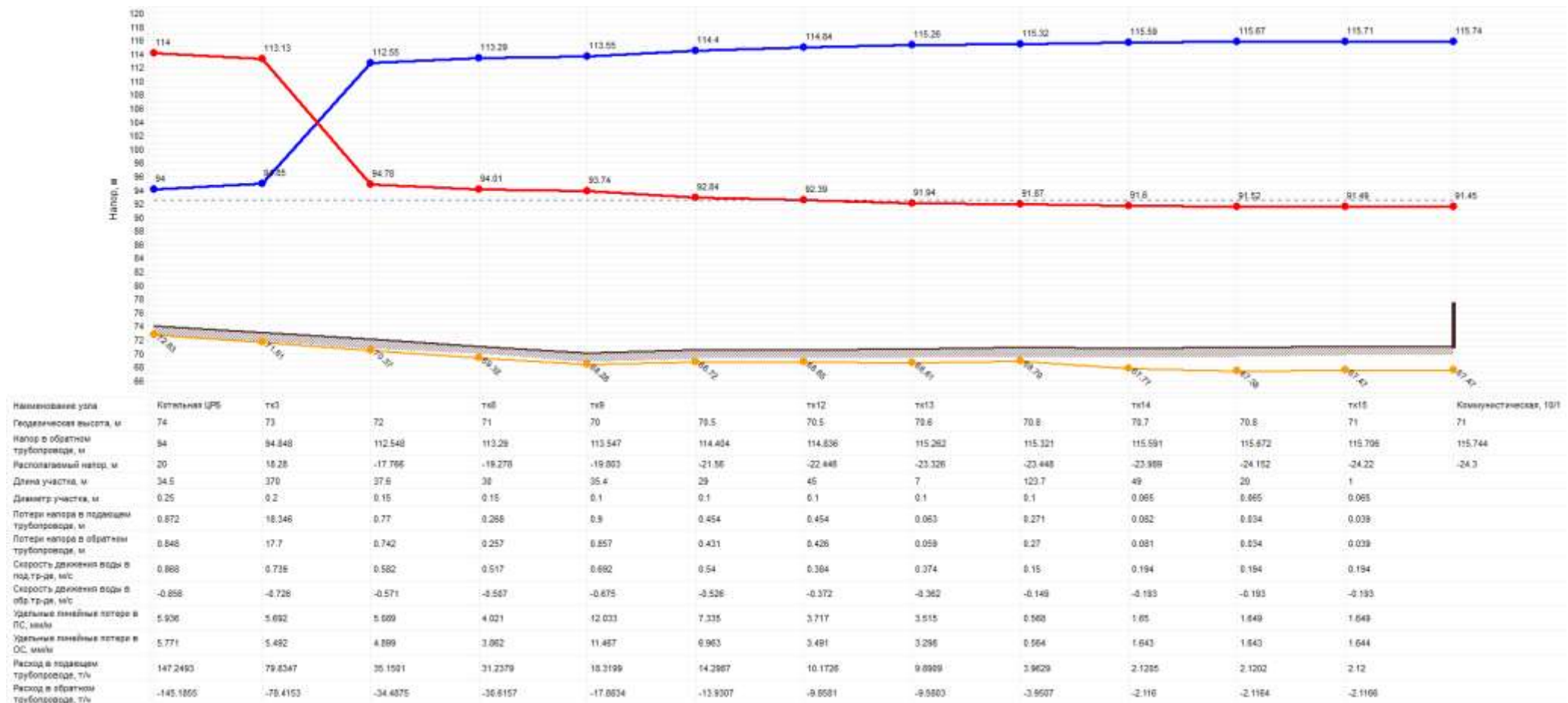
Пьезометрический график от котельной «ЦРБ» до самого удаленного потребителя.
