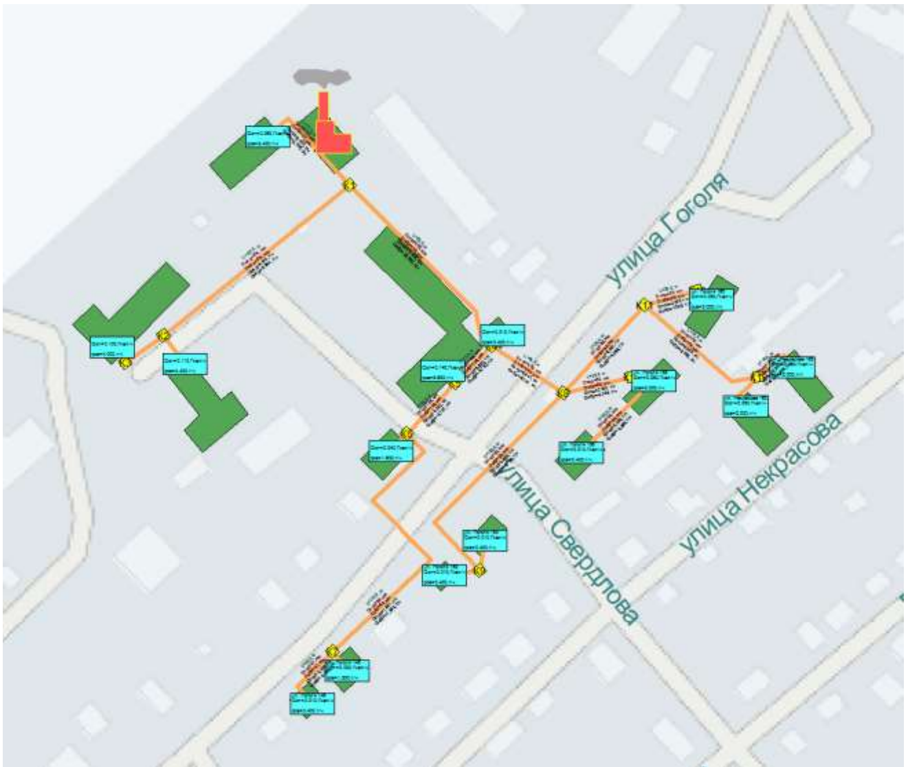
Рисунок 103. Зона действия котельной «ДРСУ».
