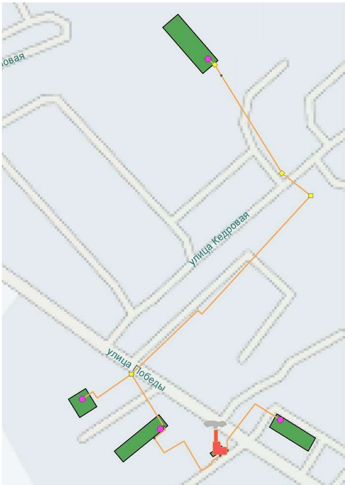
Рисунок 42. Схема тепловых сетей котельной «РММ».
